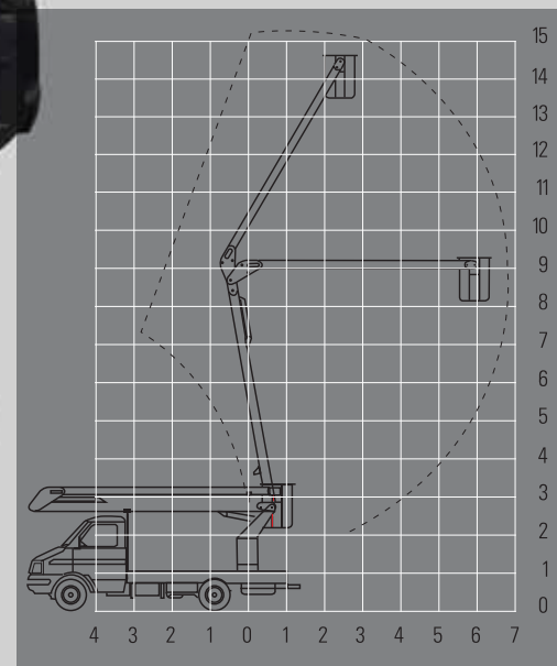
Diagrama de Alcances Hidralift 240/15
