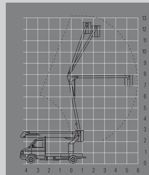
Diagrama de Alcances Hidralift 240/13
