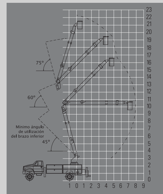
Diagrama de Alcances VAM 270/22
