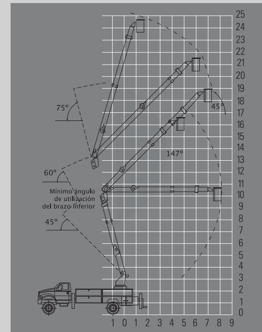
Diagrama de Alcances VAM 270/25
